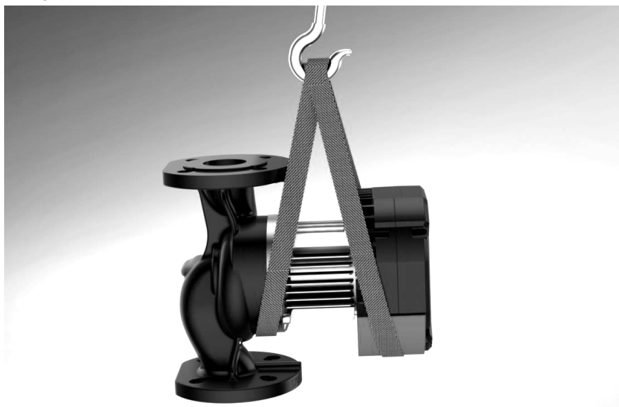
Не допустимый способ строповки насоса
